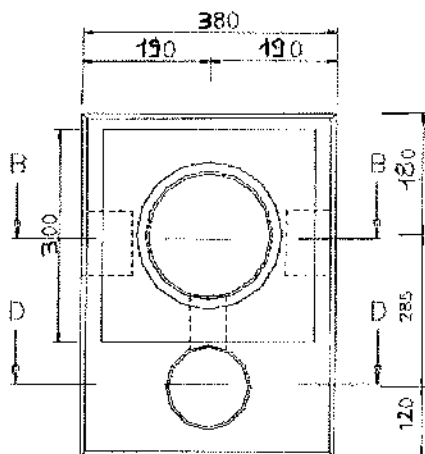
Pianta
