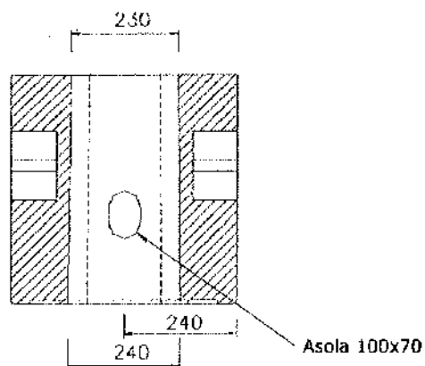
SEZIONE B-B
